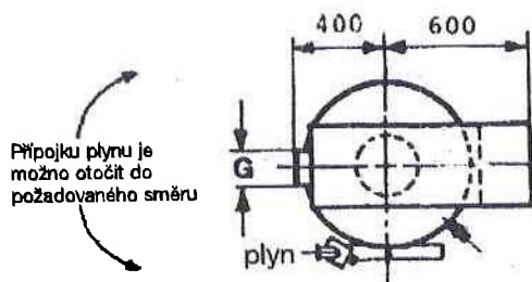
Půdorys
